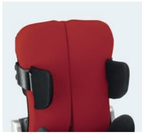
固定侧面支撑 8910401-x, 8910401-xP 高度和宽度可调整 型号 尺寸 1 W:11 x H:7 cm 2 W:10 x H:10 cm 3 W:12 x H:14 cm 4 W:16 x H:9 cm 5 W:16 x H:15 cm 6 W:12 x H:14 cm
